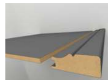
8 mm Schranktürprofil 8 mm Cabinet Door Profile
