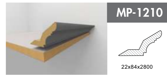
Multifunktionsprofil Multi Purpose Profile
